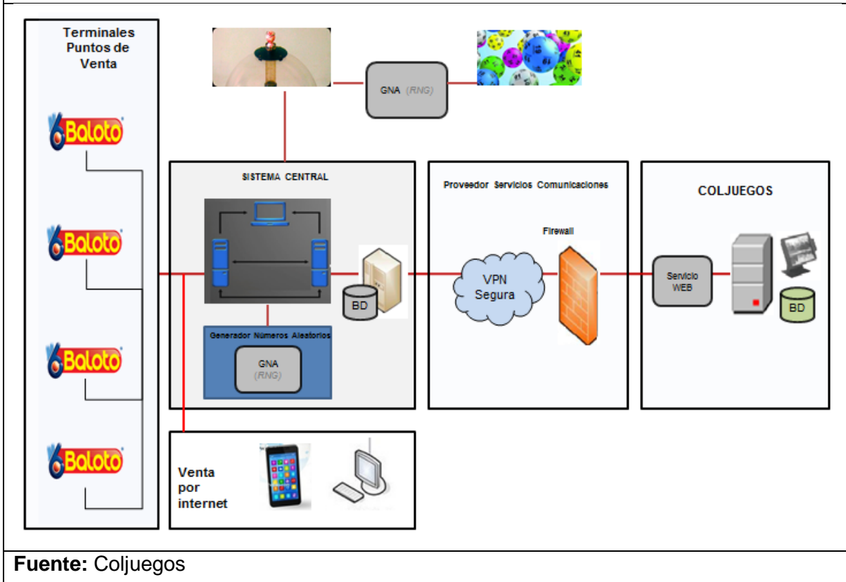
Ilustración 1. Arquitectura requerimientos técnicos BALOTO REVANCHA O CUALQUIER TIPO DE APUESTA TIPO LOTO EN LÍNEA
